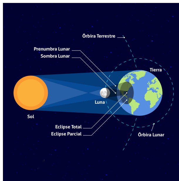
Figura 5: Zonas de umbra y penumbra en eclipse de solar
