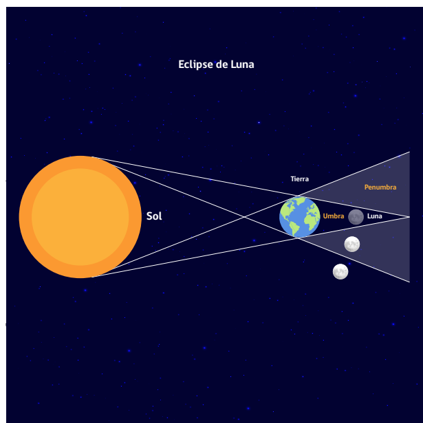
Figura 4: Zonas de umbra y penumbra en eclipse de Luna
