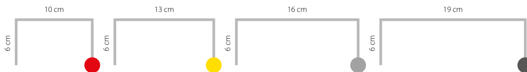
Figura 3: Alambres doblados en forma de U cuadrada y medidas en cm de cada uno. En uno de sus extremos se observan los satélites Luna Io (naranja/rojo), Luna Europa (amarillo), Luna Ganímedes (gris claro/plateado), y Luna Calisto (gris oscuro).
